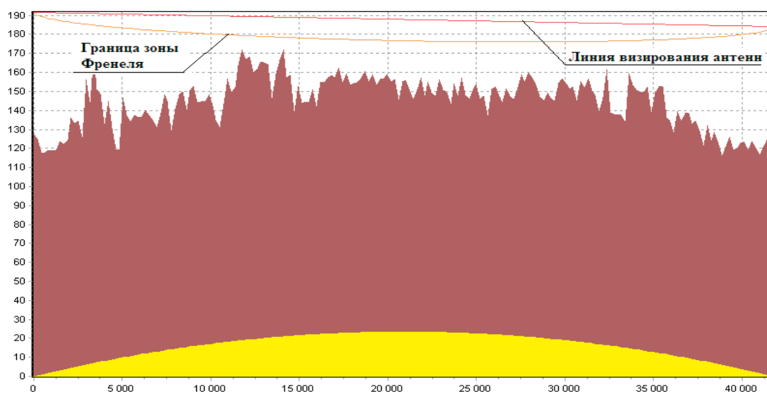
Рисунок 2а. Продольный профиль пролета А-В с учетом рельефа и подстилающей поверхности местности
