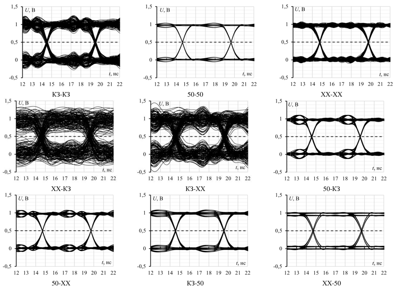
Рис. 6. Фазовые и амплитудные отклонения при различных оконечных нагрузках на концах пассивной линии
