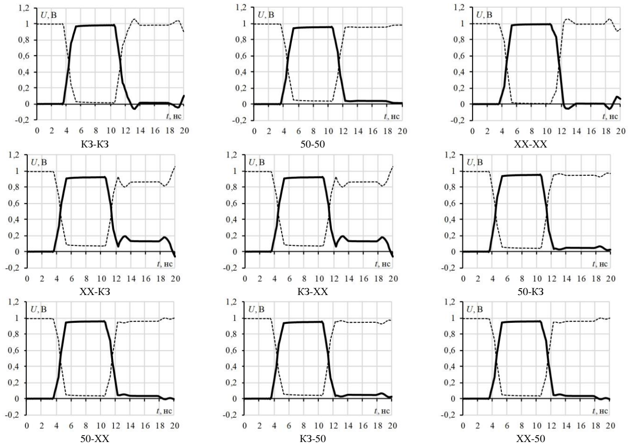
Рис. 5. Формы напряжения одиночного импульса ПСБП на выходе активной линии при различных оконечных нагрузках на концах пассивной линии
