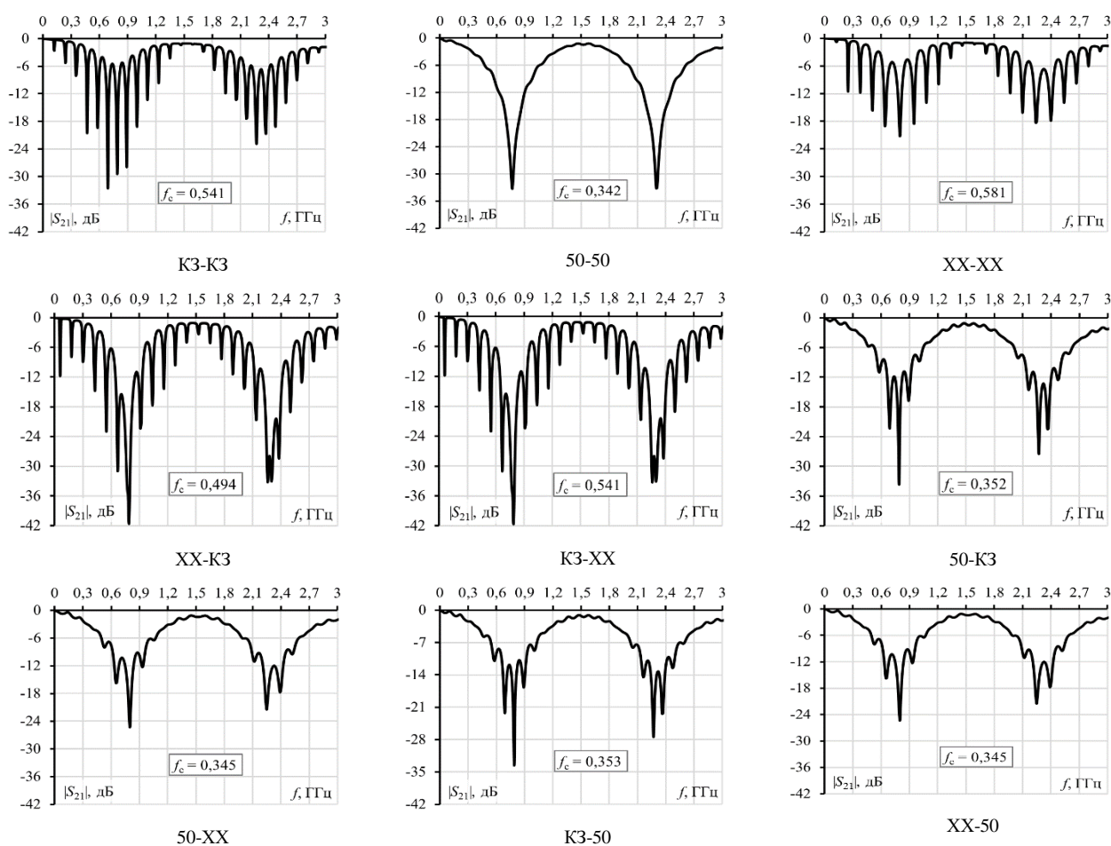
Рис. 4. Частотные зависимости |S_{21}| при различных оконечных нагрузках на концах пассивной линии
