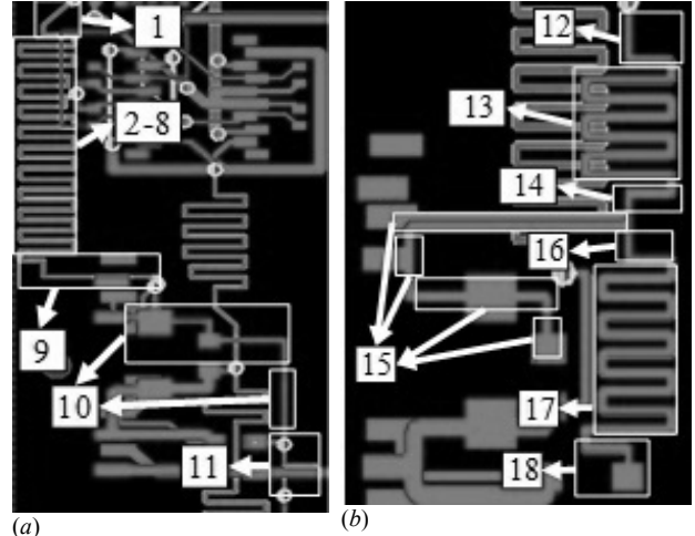
Fig. 7. Fragments of PCB: a) 1-11, b) 12-18.
