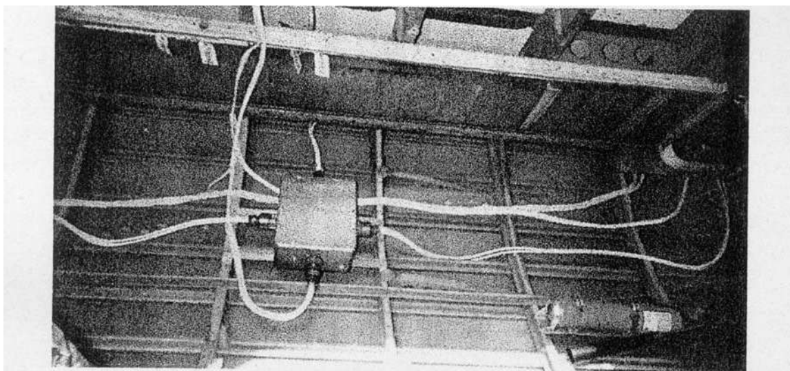
Figure III-32 : Câblage non blindé installé dans la soute avant faradisée de l'avion EMPTAC
