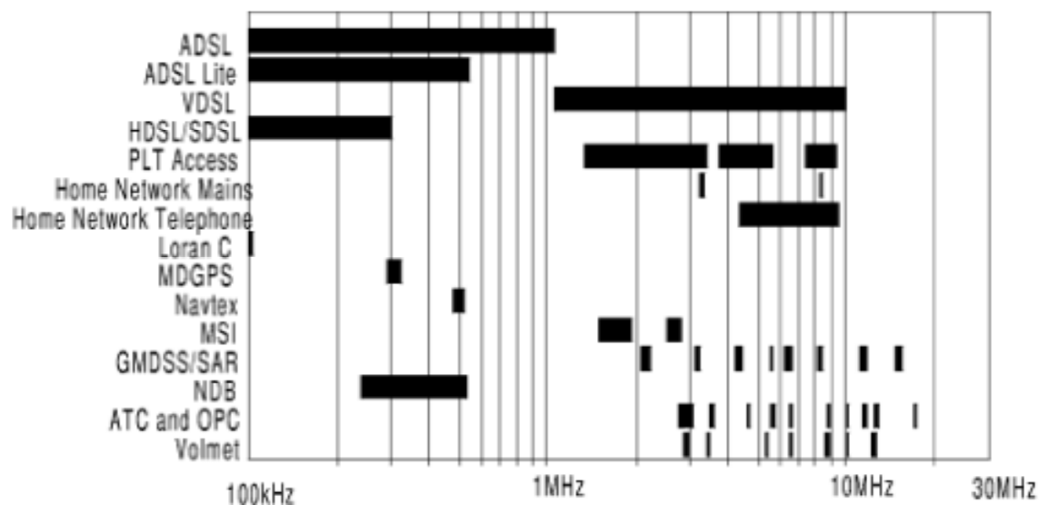
Рис. 3.11. Перекрытие частот неструктурированных сетей и морских и авиационных радиослужб
