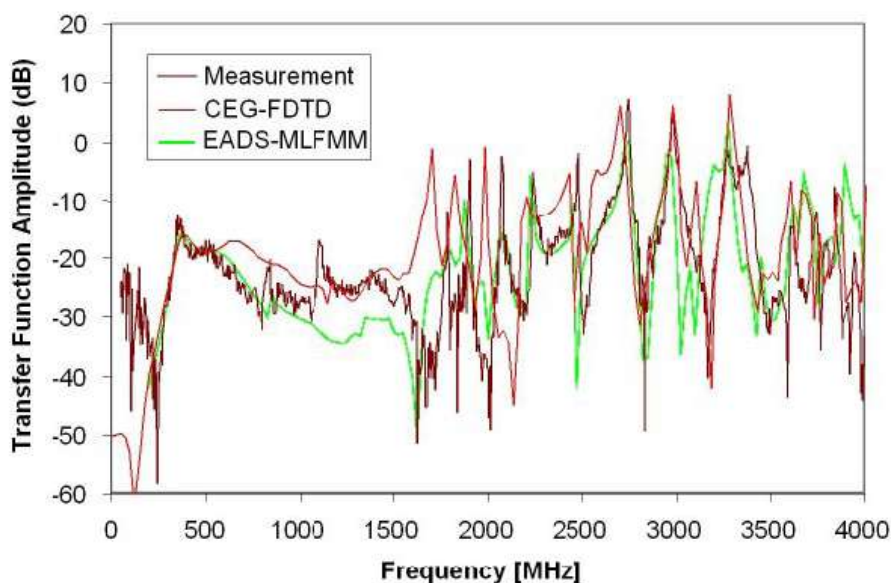
Рис. 4.10. Пример передаточной функции электрического поля для волны из свободного пространства до тестовой точки внутри GENEC. Сравнение результатов моделирования в CEG (Centre des Etudes de Gramat), кодом Protheus/MLFMA и измерений
