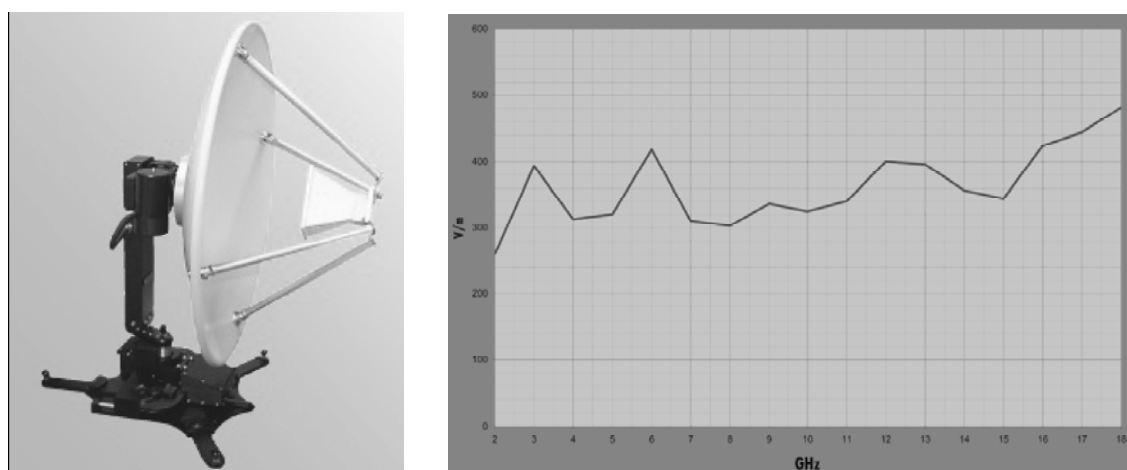
Рис. 3.8. Вид антенной системы ( a ) и типовая напряженность поля на расстоянии 1 м ( б )
