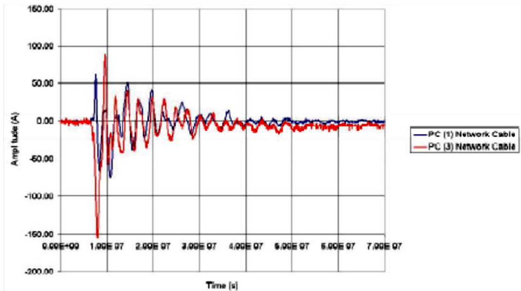
Рис. 4.2. Импульсный имитатор QinetiQ ( a ), типичный измеренный импульс поля в имитаторе ( б ), наведенные в кабелях токи при 45 кВ/м ( в ) (начало, окончание см. на с. 32)
