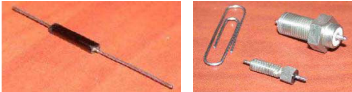
Рис. 6.11. UG-фильтр в выводном ( a ), проходном ( б ) исполнении
