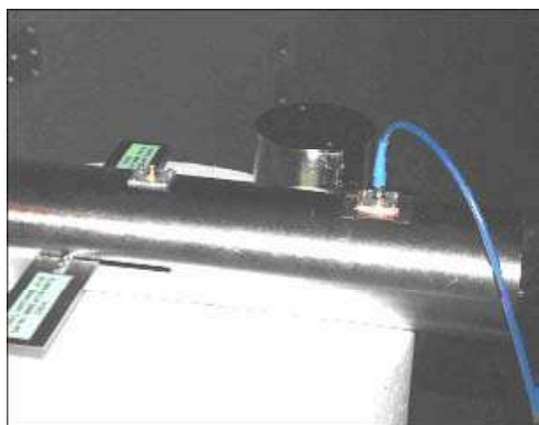
Рис. 4.8. Ракета GENEC (FOL – Fiber Optic Lead) ( a ). Крылья, щель и места двух датчиков с одним присоединенным ( б ).
