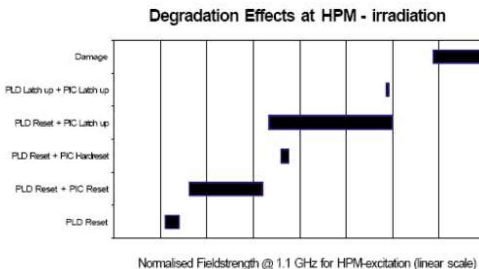
Рис. 4.11. Деградационные эффекты при воздействии мощных микроволн (начало, окончание см. на с. 42)
