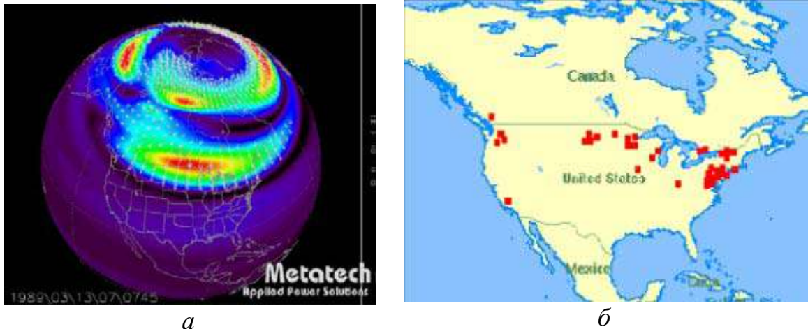
Рис. 4.13. Карта погоды, с контурами производной от магнитных полей в момент аварии сети питания (Hydro-Quebec, 7:45 UT or 2:45 EST, March 13, 1989) (а). Зафиксированные влияния на сеть питания в Северной Америке, March 13, 1989, time 16:00–17:23 EST (21:00–22:23 UT) (б)
