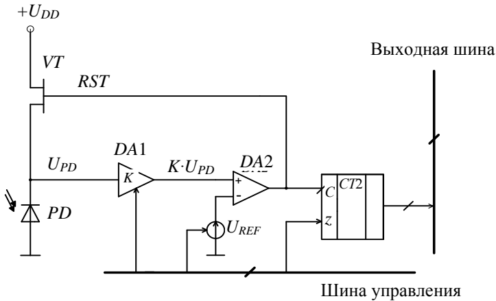
Рис. 4.3.2. Цифровой пиксел с преобразованием сигнал-частота и регулируемым размером групп фотогенерированных электронов (регулируемым коэффициентом усиления)
