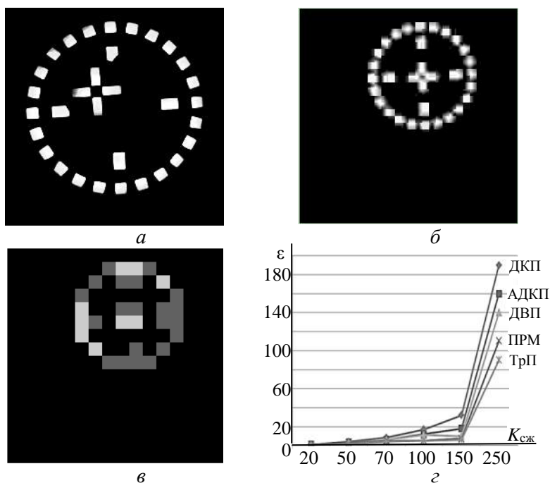
Рис. 2.3.9. Фрагмент кадра с изображением мишени: при сжатии меньше критического – а ; при критическом сжатии – б ; при сжатии более критического – в ; и зависимость ошибки измерения промаха от коэффициента сжатия при различных алгоритмах кодирования – г
