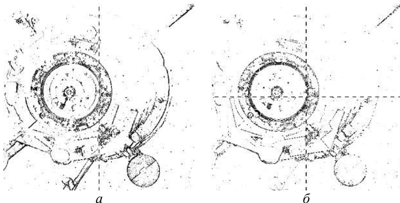
Рис. 2.3.6. Изображение КА (см. рис. 2.4.1): после межэлементного вычитания ( D_{\Delta x} = 78 ) – а; после двумерной фильтрации ( D_{\Delta xy} = 22 ) – б
