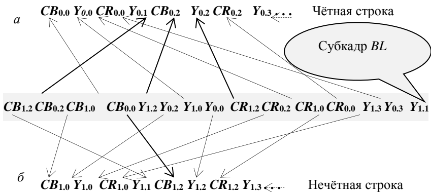
Рис. 3.3.14. Схема компоновки субкадров из отсчётов параллельного мультиплекса
