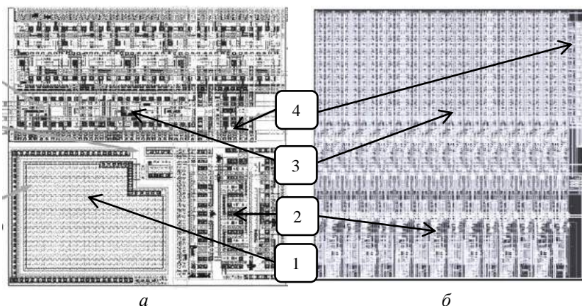
Рис. 4.3.3. Топология цифрового пиксела при засветке: прямой – a ; обратной – б (фотодиод сформирован по всей площади пиксела с обратной стороны кристалла); 1 – фотодиод, 2 – компаратор, 3 – счётчик, 4 – узел управления
