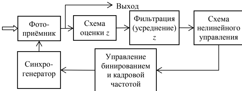
Рис. 2.4.4. Структура системы с адаптивным управлением
