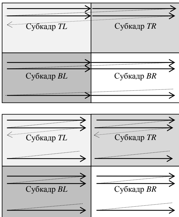
Рис. 3.3.13. Порядок буферизации субкадров: а – очередность последовательной записи отсчётов в буферы; б – очередность параллельного считывания отсчётов из буферов
