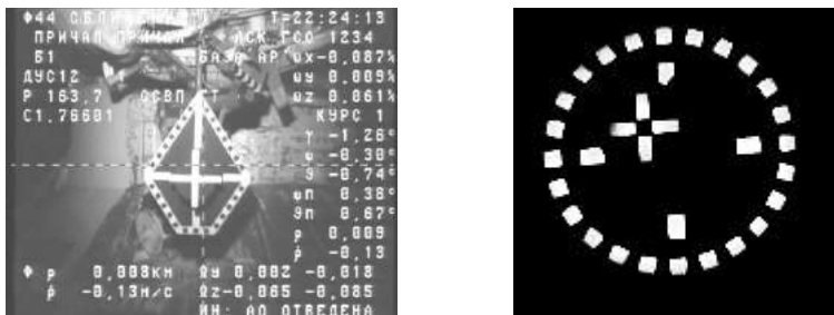
Рис. 3.4.2. Объемные реперы позволяют по смещению малого и большого перекрестий измерить отклонение стыковочных узлов кооперируемых КА
