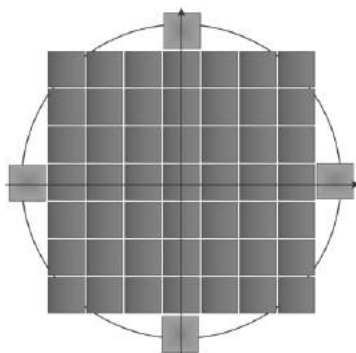
Рис. 4.4.4. Схема фокальной сборки из 49 матриц и её параметры
