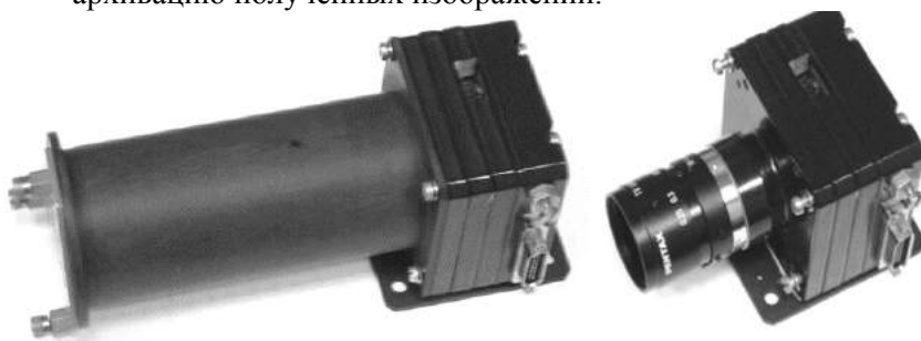
Рис. 3.2.9. ТВ камера звёздного датчика с блендой и без бленды
