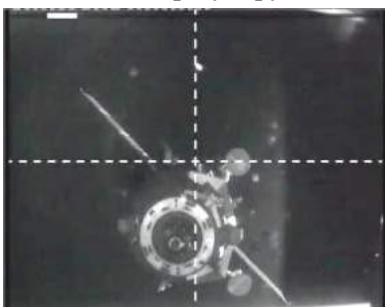
Рис. 3.2.13. Сложные световые условия наблюдения: бликовая ситуация – а; неравномерность подсветки – б
