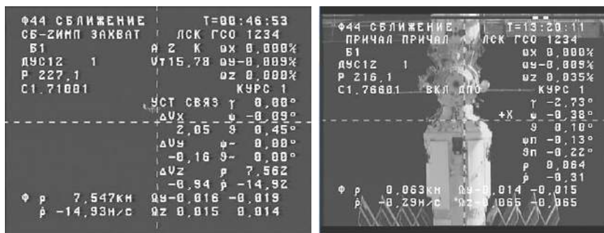
Рис. 3.4.22. Изображение МКС, переданное с транспортного корабля в ходе сближения на дистанциях 7,5 км и 0,06 км
