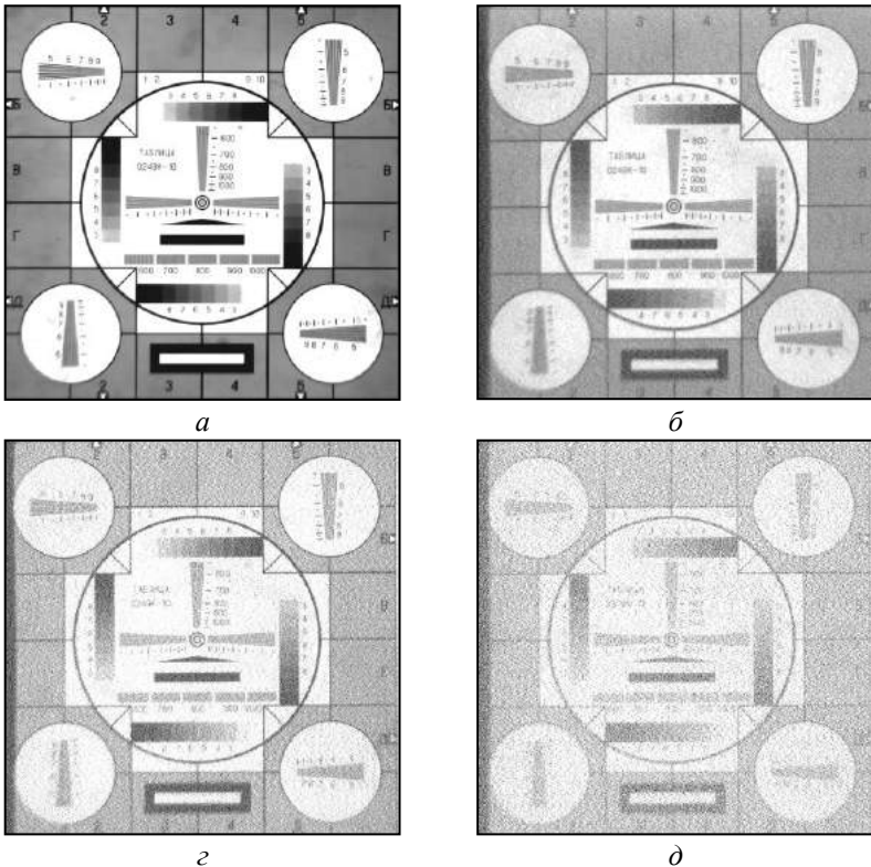
Рис. 3.2.10. Примеры изображений, формируемых ТВ камерой звёздного датчика при лабораторных испытаниях
