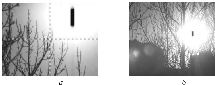
Рис. 3.2.15. Искажения изображения при попадании Солнца в поле зрения ТВ камеры на КМОП фотоприёмной матрице: узкоугольной – а ; широкоугольной – б
