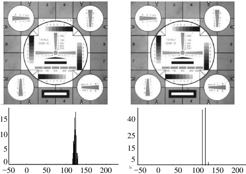
Рис. 2.3.1. Изображение тест-таблицы (вверху); гистограммы шума на уровне серого (внизу); квантование избыточное, Q = 0,7 \times 10^6 (слева) и оптимальное Q = 1,8 \times 10^6 (справа)
