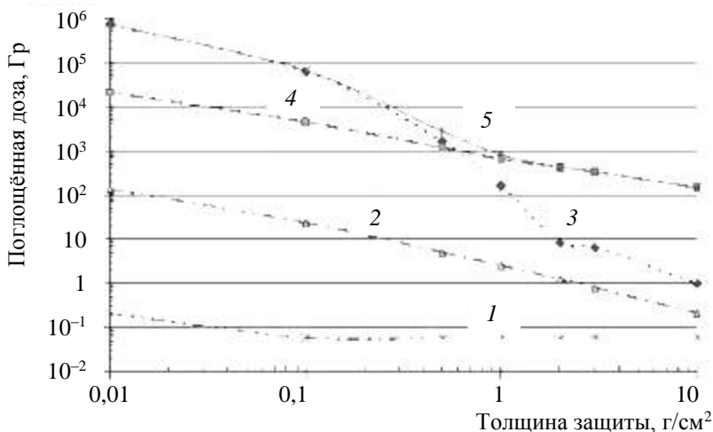
Рис. 3.1.3. Зависимость поглощённой дозы за 5 лет эксплуатации на орбите 1 – галактические космические лучи; 2 – солнечные космические лучи; 3 – электроны радиационных поясов Земли; 4 – протоны радиационных поясов Земли; 5 – суммарная доза
