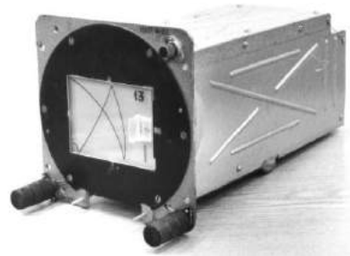
Рис. 1.2.21. Индикатор (ВКУ) КР-73А с «маской» из комплекса ТВ-аппаратуры КЛА Л1
