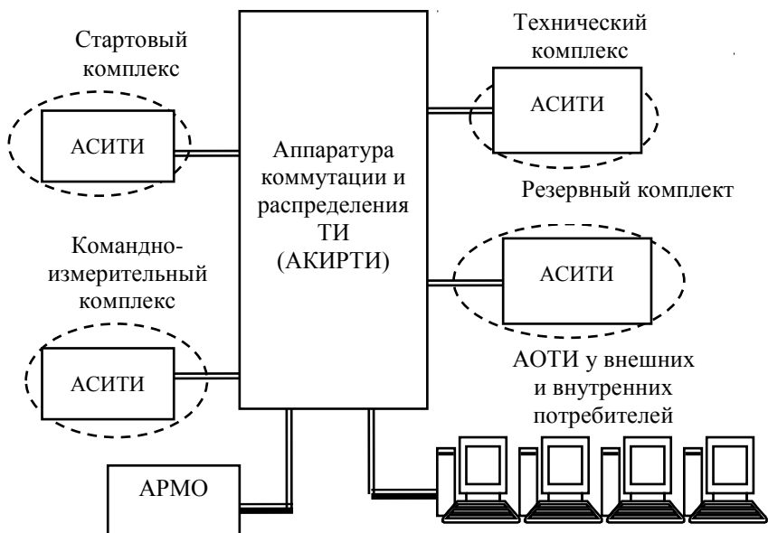
Рис. 3.9.2. Структурная схема ЦКК и РТИ
