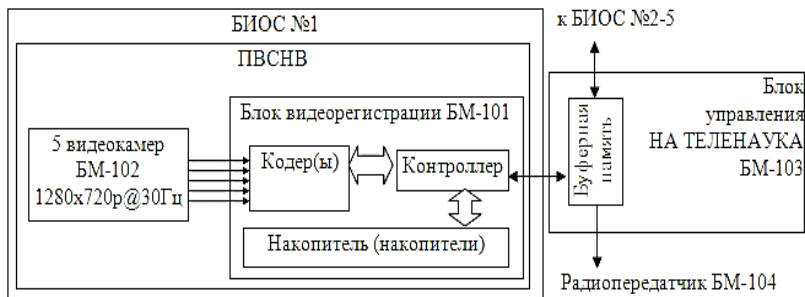
Рис. 3.5.2. Архитектура видеоканала НА «Теленаука»
