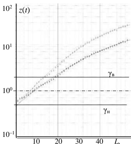
Рис. 2.4.9. Изменение статистики z_k в ходе сближения КА; точки – эксперимент, кривые – аппроксимация \varphi(k) ; внизу – полное разрешение, вверху – бининг 2 \times 2
