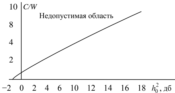
Рис. 2.5.1. Зависимость пропускной способности в полосе канала от ОСШ
