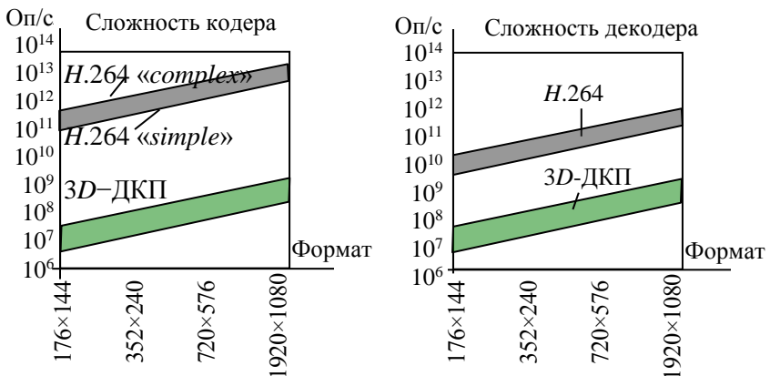
Рис. 2.3.14. Зависимость сложности кодирования и декодирования от формата кадра
