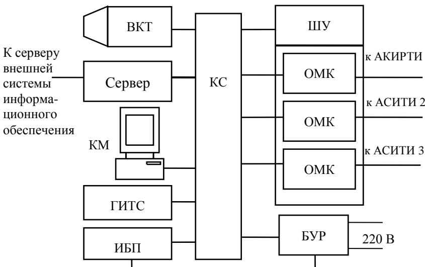
Рис. 3.9.3. Структурная схема АСИТИ
