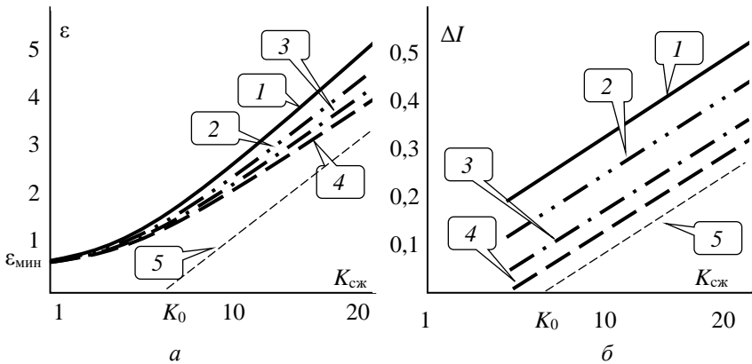
Рис. 2.3.10. Зависимость ошибки (а) и потери информации (б) от сжатия для: ДКП – 1; ДВП – 2; ДПП – 3; ТрП – 4; и предел – 5, определяемый соотношением энтропии источника и пропускной способности
