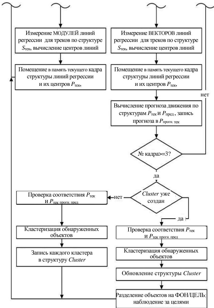
Рис. 2.2.5. Алгоритм совместного обнаружения–оценивания на основе измерения авторегрессии и межкадровой обработки при формировании кластеров
