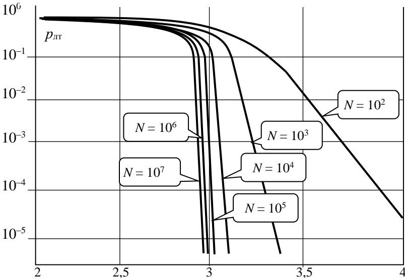
Рис. 2.4.12. Зависимость вероятности превышения порога \gamma_{\text{в}} статистикой z при \varphi = 2 для выборок объёмом N = 10^2 \dots 10^7
