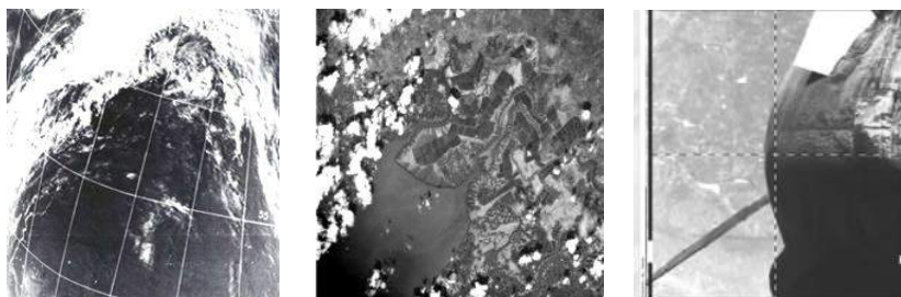
Рис. 2.1.5. Изображения, полученные из космоса, при оптическом контрасте более 4 порядков
