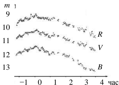
Рис. 2.2.12. Изменения во времени видимого блеска ИСЗ «Интелсат-4», полученные квазиодновременно в полосах B , V , R согласно [142], [143]
