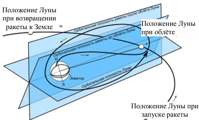
Рис. 1.2.3. Траектория полёта автоматической станции «Луна-3»
