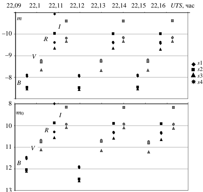
Рис. 2.2.18. Результаты обработки наблюдений с фильтрами; инструментальные звёздные величины m (вверху), вычисленные с использованием звёздного каталога значения m_0 (внизу); разные виды значков соответствуют разным спутникам
