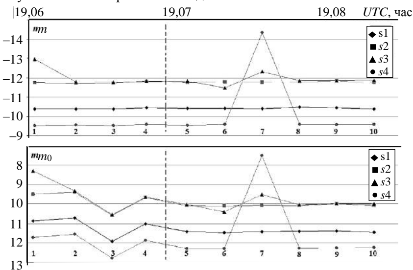
Рис. 2.2.14. Результаты наблюдения четырёх ИСЗ: инструментальные звёздные величины m (вверху), вычисленные с использованием звёздного каталога значения m_0 (внизу); по оси абсцисс – время съёмки кадров; вертикальная пунктирная линия отделяет кадры, снятые без часового ведения (1–4), от кадров с часовым ведением (5–10)
