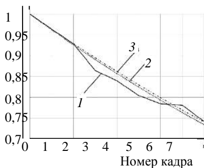
Рис. 2.1.14. Измеренная АКФ по времени сюжета рис. 2.1.9а — 1; её аппроксимация для марковского процесса 1-го порядка — 2 (СКО 0,103); аппроксимация для марковского процесса 2-го порядка — 3 (СКО 0,107)
