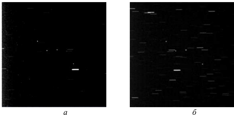
Рис. 2.2.17. Изображения спутников и смазанных звёзд при наблюдении: с фильтрами B – a ; с фильтрами I – b
