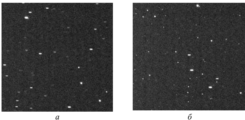
Рис. 2.2.13. Изображения звёзд и спутников: в режиме слежения за спутниками, изображения звёзд смазаны – а ; в режиме слежения за звёздами, изображения спутников смазаны – б
