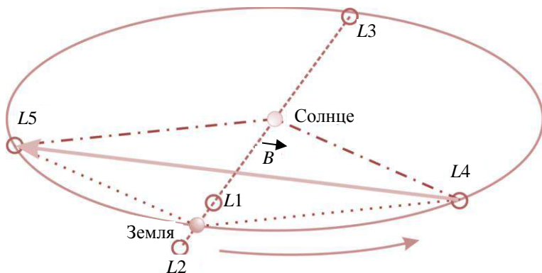
Рис. 4.4.3. Два КА расположены в западной L_4 и восточной L_5 точках, положение которых определяется текущим положением Земли в орбите
