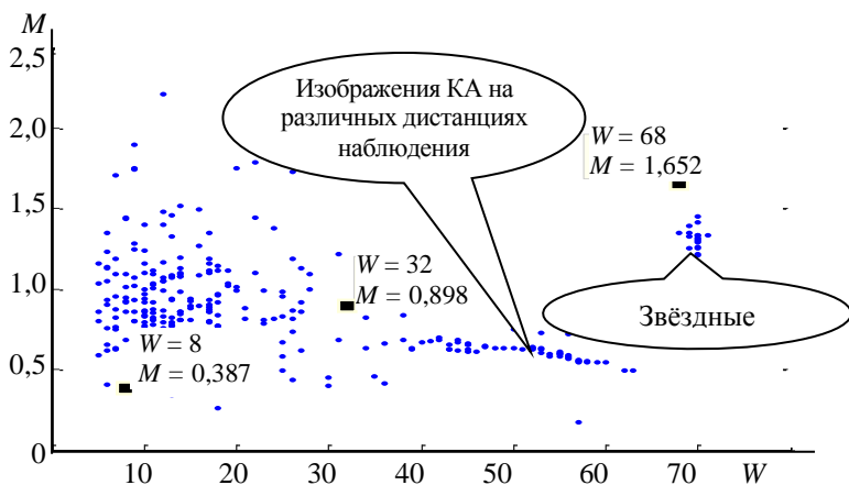
Рис. 2.1.6. Значения мер широкополосности W и нестационарности M по полю для избыточной выборки сюжетов
