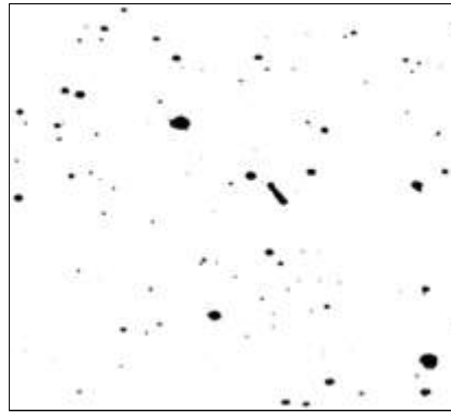
Рис. 2.2.2. Неподвижное поле звёзд и подвижный объект (негатив)
