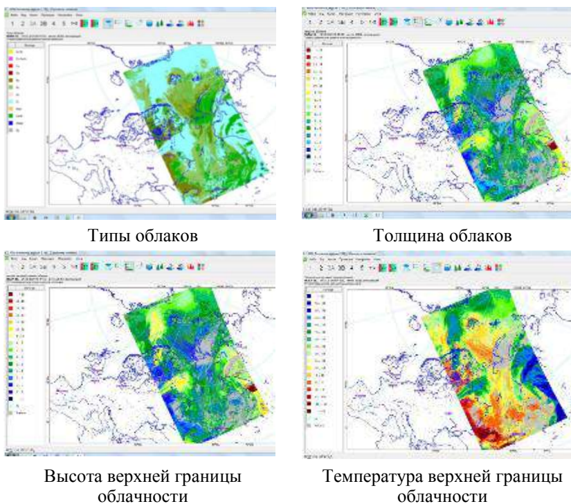
Рис. 3.7.7. Результаты тематической обработки спутниковой метеоинформации – карты параметров облачности над севером Евразии
