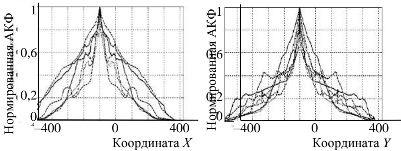
Рис. 2.1.10. Семейство пространственных корреляционных функций
