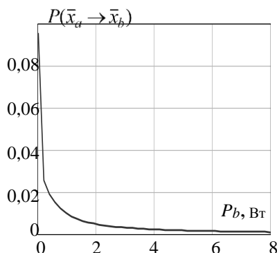
Рис. 2.5.23. Зависимость вероятности парной ошибки от значения мощности ВСС P_b
