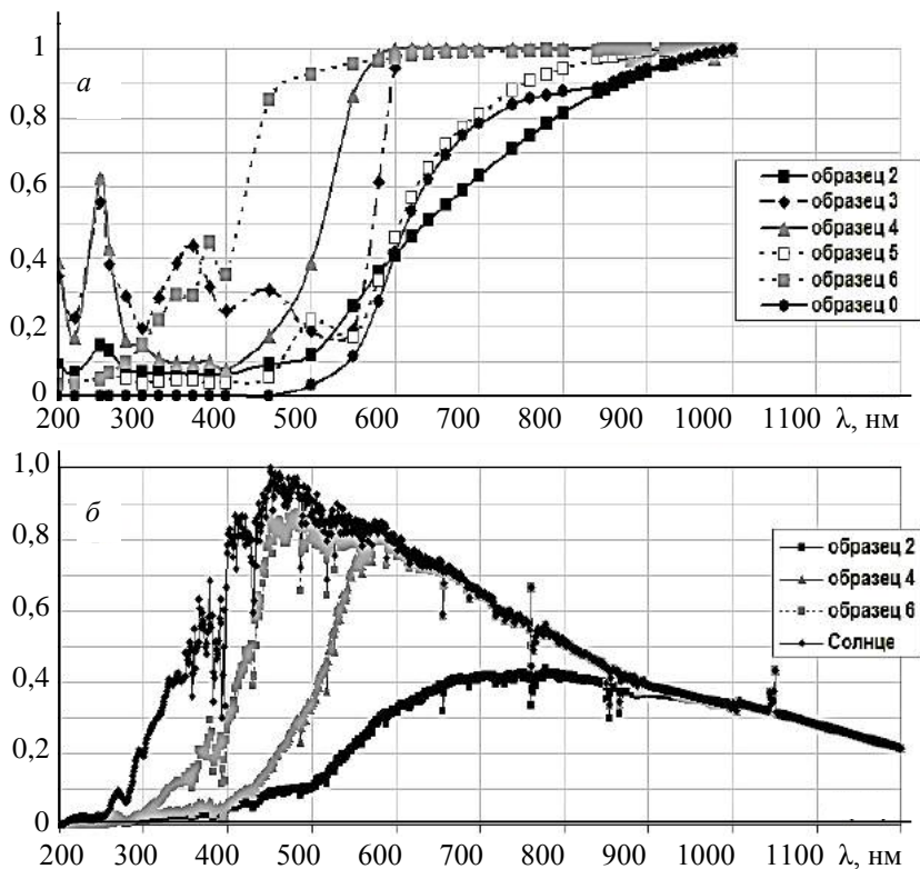
Рис. 2.2.19. Нормированные спектры отражения образцов ЭВТИ – а; спектры отражения ими излучения Солнца – б
