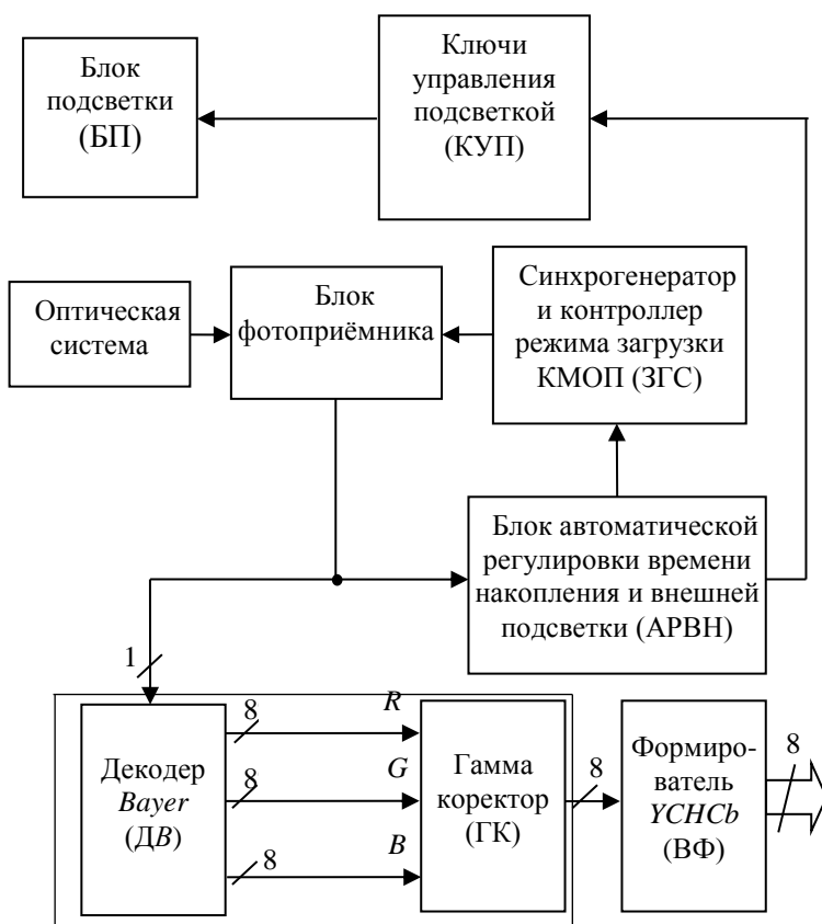
Рис. 3.5.2. Структурная схема телевизионной системы Орлан-2
