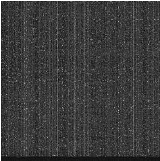
Рис. 3.1.7. Темновой сигнал после воздействия облучения протонами с энергией 1 ГэВ при дозе, эквивалентной 8 годам эксплуатации ТВ камеры в космосе: матрица 1 мегапиксел – а ; фрагмент матрицы с сигналом тестового объекта – б
