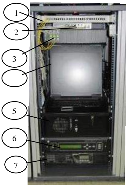
Рис. 3.9.4. Внешний вид стойки АСИТИ
