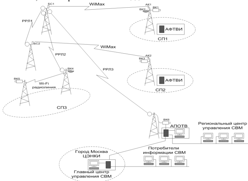
Рис. 3.9.12. Схема организации системы видеомониторинга
