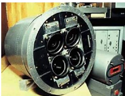
Рис. 1.2.10. Первая четырёхканальная видиконная метеорологическая система; музей НИИ телевидения
