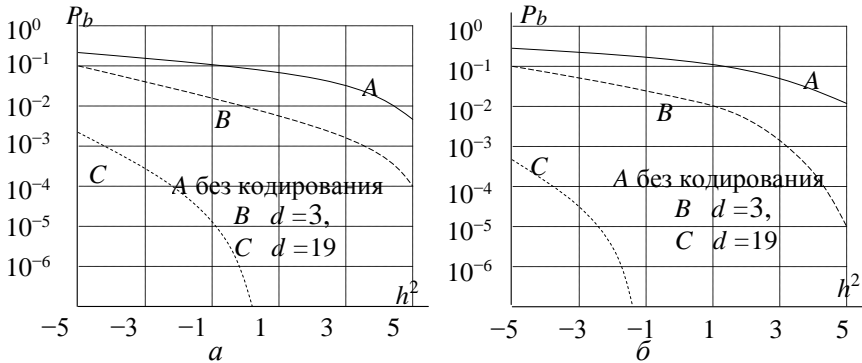
Рис. 2.5.18. Оценка характеристик оптимального декодирования СОК и для различных значений d в: ДСК – а; АБГШ – б
