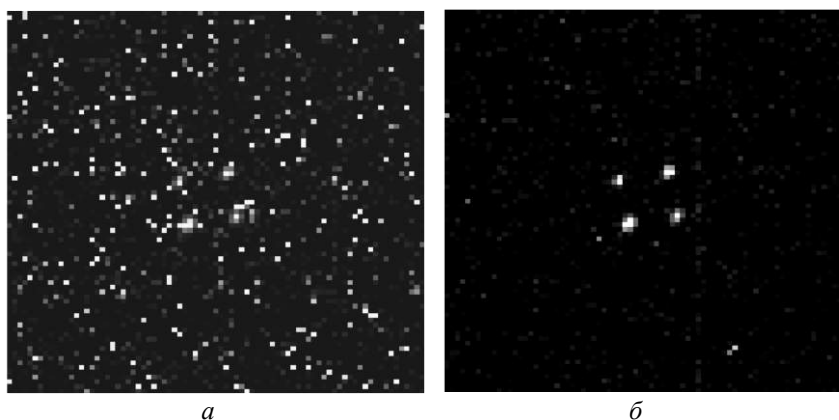
Рис. 3.1.12. Тестовый сигнал на фоне стационарных радиационных помех: после подавления столбцовых дефектов с помощью метода (3.2) – а ; после подавления стационарных точечных дефектов межкадровой обработкой – б
