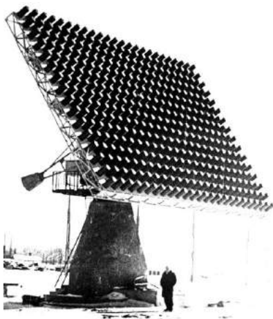
Рис. 1.2.15. Антенна для связи наземного пункта с КА
