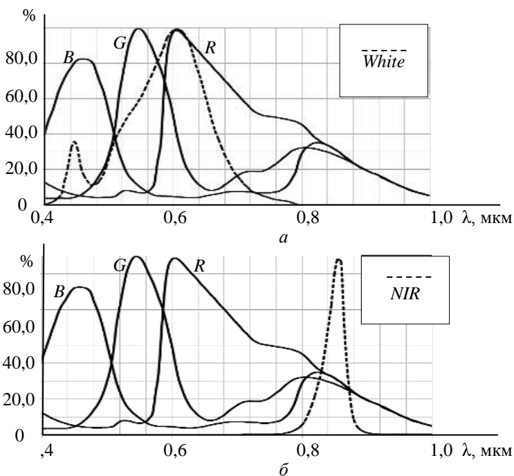
Рис. 3.5.4 Спектральные характеристики цветodelённых каналов и светодиодов подсветки в режиме: «день» – a ; «ночь» – б
