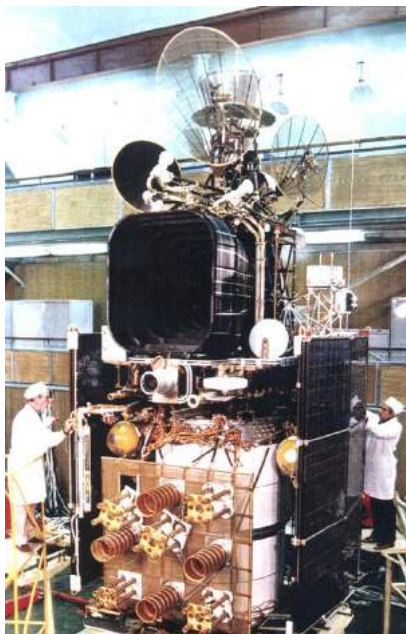
Рис. 1.2.14. Сборка КА «Электро» с аппаратурой «Метеорит-Планета»
