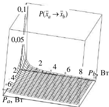
Рис. 2.5.24. Зависимость вероятности парной ошибки от взаимных значений мощностей ВСС P_a и P_b
