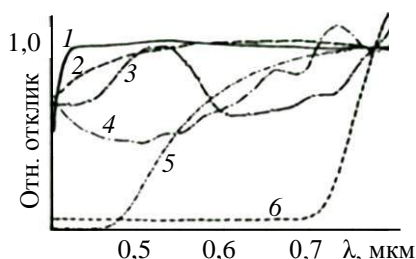
Рис. 2.2.10. Относительные спектральные характеристики отражения различных покрытий 1 согласно [140]
