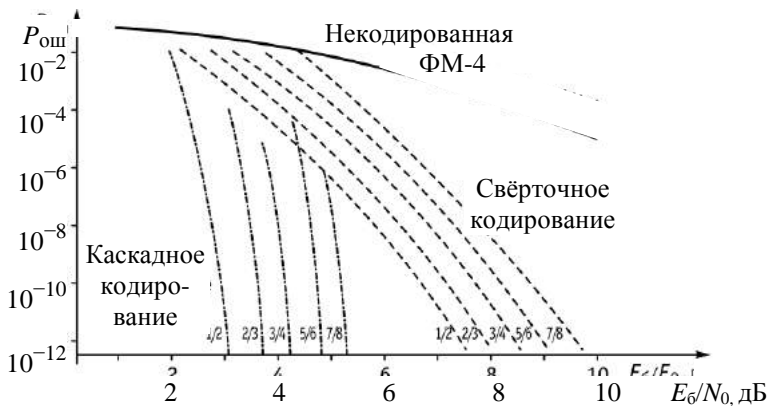
Рис. 2.5.12. Зависимости вероятности ошибки P_{\text{ош}} от отношения E_b/N_0 для QPSK -модуляции при разных относительных скоростях кодирования
