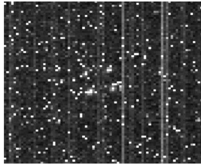
Рис. 3.1.7. Темновой сигнал после воздействия облучения протонами с энергией 1 ГэВ при дозе, эквивалентной 8 годам эксплуатации ТВ камеры в космосе: матрица 1 мегапиксел – а ; фрагмент матрицы с сигналом тестового объекта – б
