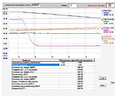
Рис. 3.9.27. Скриншот изображения телеметрического формуляра, получаемого от ВКИП
