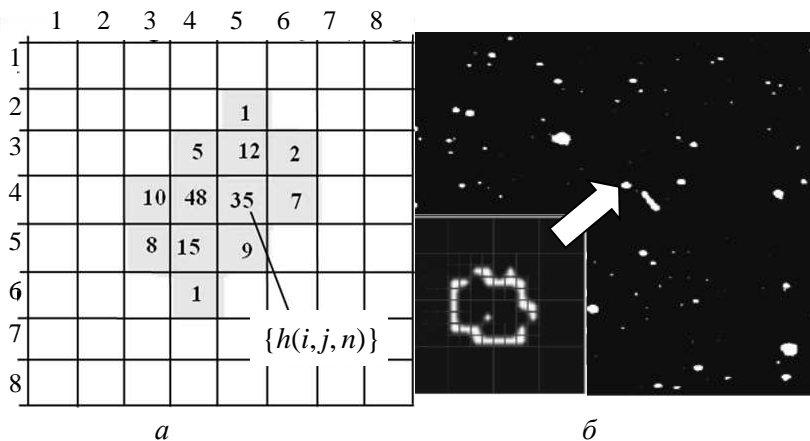
Рис. 2.2.3. Изображение объекта в уровнях яркости его элементов – а; результат выделения одного из объектов (одной из связанных областей) – б
