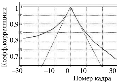
Рис. 2.1.11. Временная АКФ сюжета рис. 2.1.9б; пунктиром показана линейная аппроксимация АКФ, оптимальная для малых абсолютных значений аргумента
