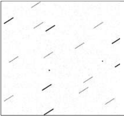
Рис. 2.2.1. Подвижное поле звёзд и неподвижные объекты (негатив)
