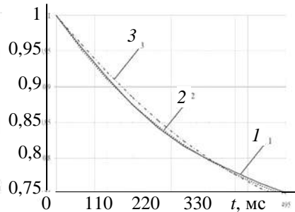
Рис. 2.1.12. Измеренная АКФ по времени сюжета рис. 2.1.9б 1, её аппроксимация для марковского процесса 1-го порядка 2 (СКО 0,019), аппроксимация для марковского процесса 2-го порядка 3 (СКО 0,060)
