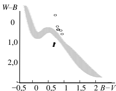
Рис. 2.2.11. Распределение колор-индексов космических объектов (кружки), покрытых различными типовыми материалами, и звёзд главной последовательности [118]
