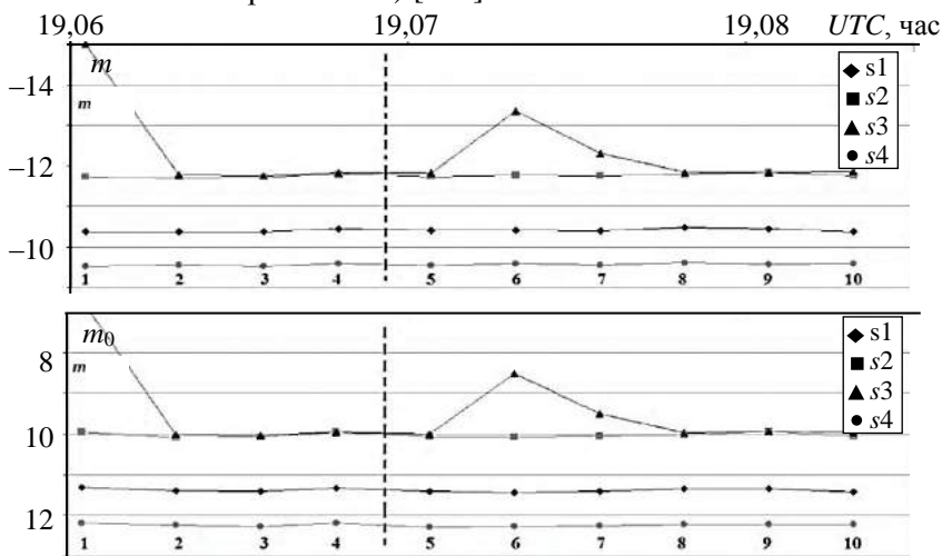
Рис. 2.2.15. Результаты наблюдения четырёх ИСЗ: инструментальные звёздные величины m (вверху), вычисленные с использованием звёздного каталога значения m_0 (внизу) (модифицированный алгоритм измерения треков)
