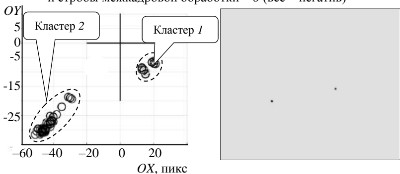
Рис. 2.2.7. Разделение обнаруженных сигналов на кластеры по вектору смаза
