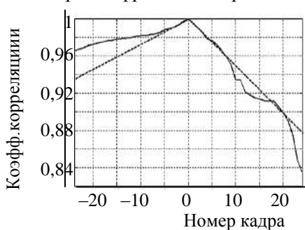
Рис. 2.1.13. Временная АКФ сюжета рис. 2.1.9а; пунктир — линейная аппроксимация АКФ, оптимальная для малых абсолютных значений аргумента
