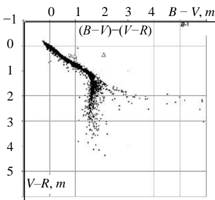
Рис. 2.2.20. Двумерная диаграмма (B-V) - (V-R) ; чёрные точки – звёзды из каталога [117], квадраты – наблюдаемые геостационарные ИСЗ, треугольники – образцы покрытий
