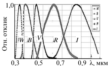
Рис. 2.2.9. Спектральные характеристики оптических фильтров фотометрической системы Джонсона по [117], [147], [148]
