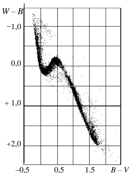
Рис. 2.1.18. Распределение колор-индексов звёзд Каталога
