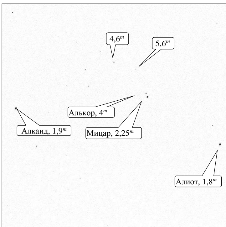
Рис. 3.2.11. Изображение участка звёздного неба (часть созвездия Большой Медведицы, негатив)
