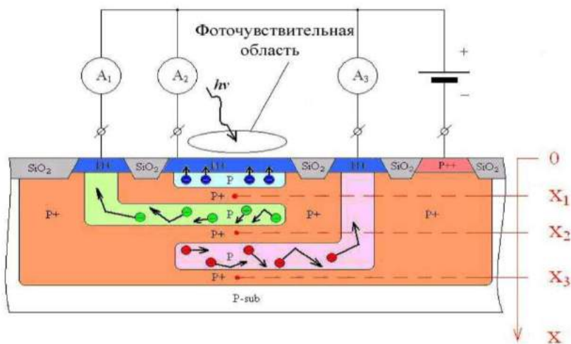
Рис. 4.3.5. Разрез фотоприёмной структуры с внутренним цветоделением: STI – поверхностная изоляция \text{SiO}_2 ; NP – зона легирования канала сбора поверхностных носителей; PP – зона легирования контакта к охранной зоне пиксела; PW – легирование охранной зоны по границе пиксела; SBB – зона легирования барьера между средними и глубокими носителями; NM – легирование канала сбора средних носителей
