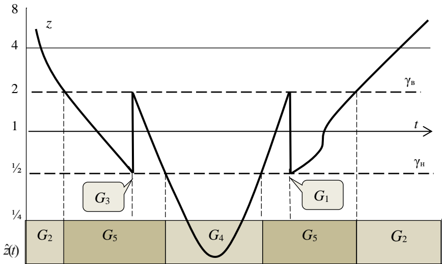
Рис. 2.4.6. Изменение состояний адаптивной телевизионной системы при изменении опорной статистики z во времени
