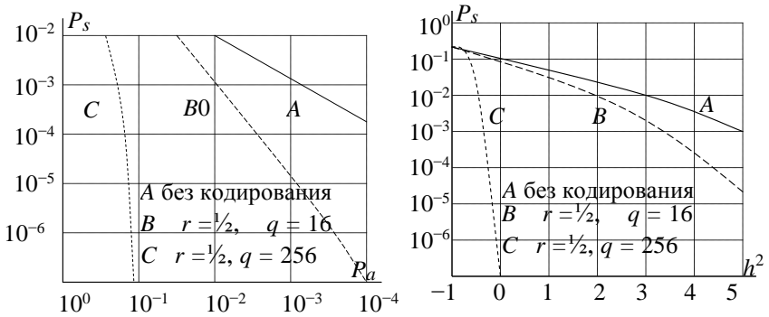
Рис. 2.5.15. Оценка характеристик КРС в q -ичном симметричном канале
