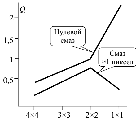
Рис. 2.3.5. Зависимость качества информации от бинирования при скоростном смазе изображения, E \approx E_{нас}
