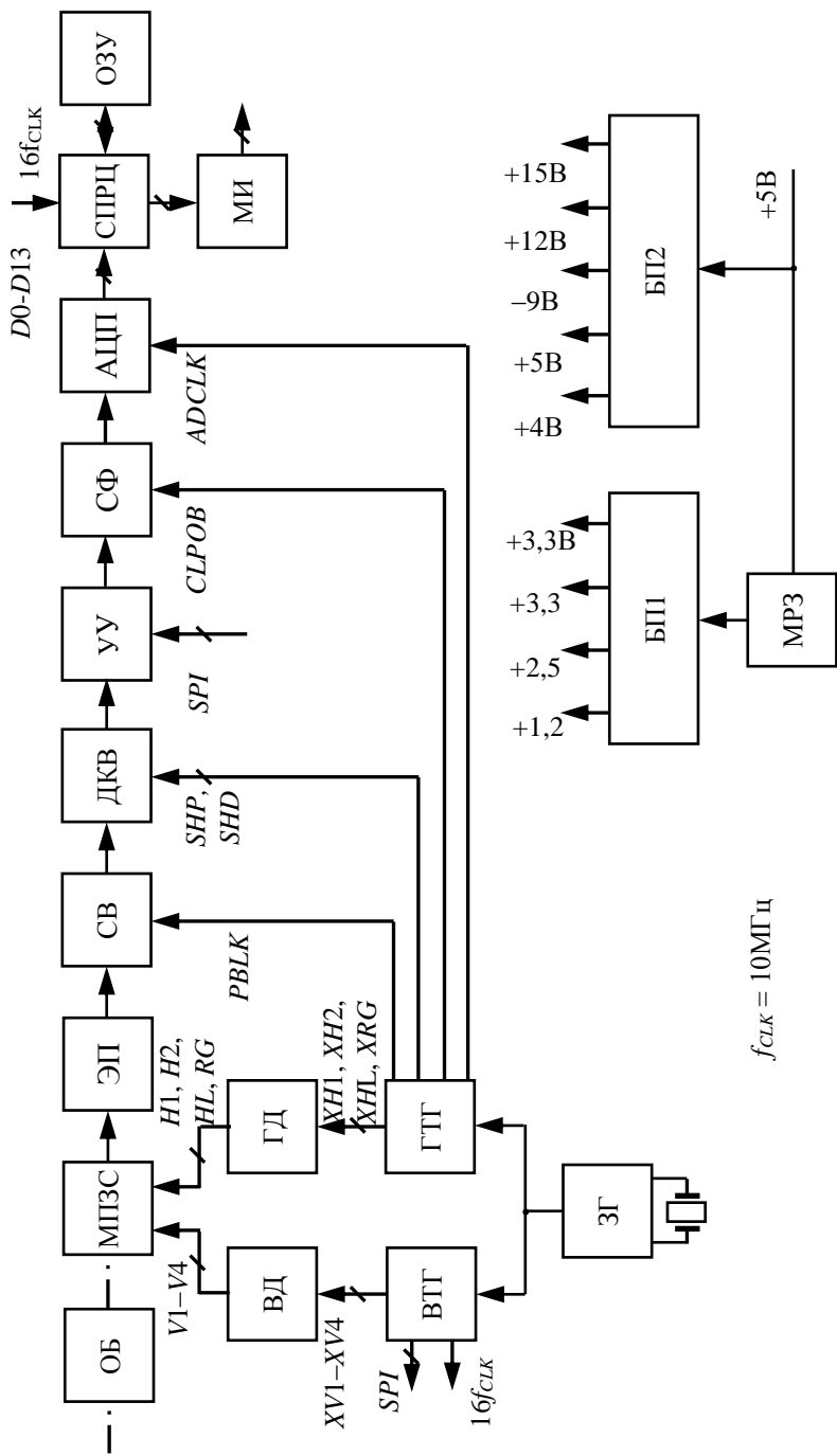
Рис. 3.2.8. Функциональная схема ТВ камеры звёздного датчика
