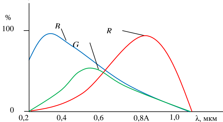
Рис. 4.3.5. Относительные спектральные характеристики матрицы
