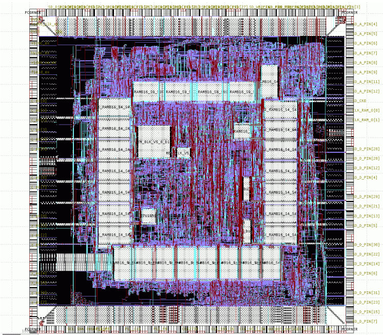
Рис. 3.3.8. Топология кодера 5022BX014
