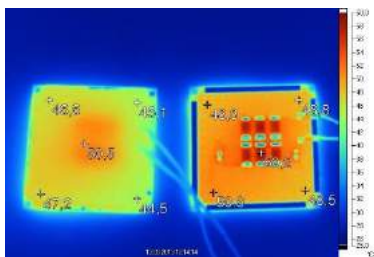
Рис. 3.1.1 Тепловые испытания компаундов вакуумной защиты
