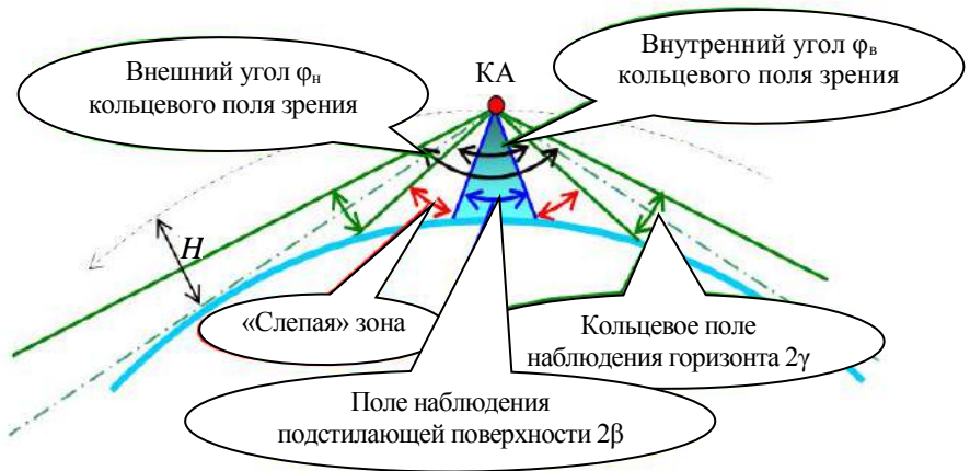
Рис. 4.3.7. Схема одновременного наблюдения подстилающей поверхности Земли и горизонта
