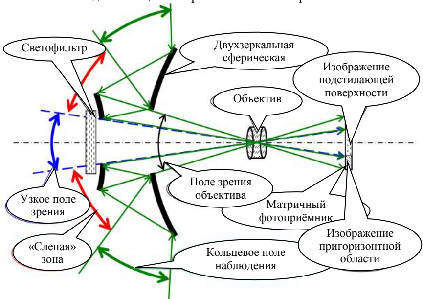
Рис. 4.3.8. Оптическая схема с коаксиально расположенными широкоугольной и узкоугольной оптическими системами
