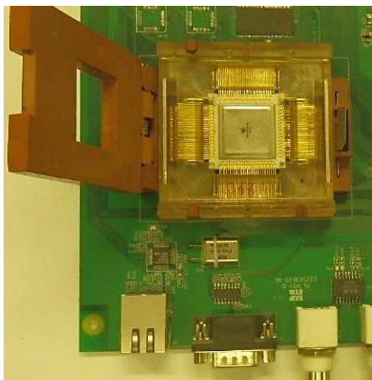
Рис. 3.3.7. EVC -кодер ( а ) и входящая в его состав микросхема 5022ВХ014 ( б )
