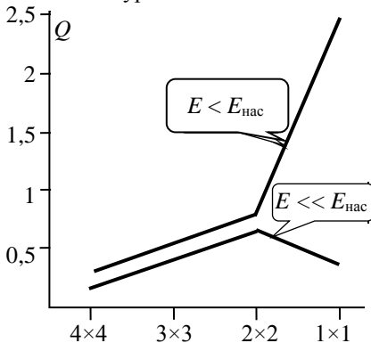
Рис. 2.3.4. Зависимость качества информации от бинирования при различных освещённости
