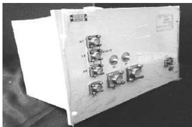
Рис. 3.4.16. Кодер КЛ-211-2
