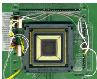
Рис. 3.2.17. Макетный образец ТВ камеры на КМОП матрице 1205XB014 формата 1024×1024
